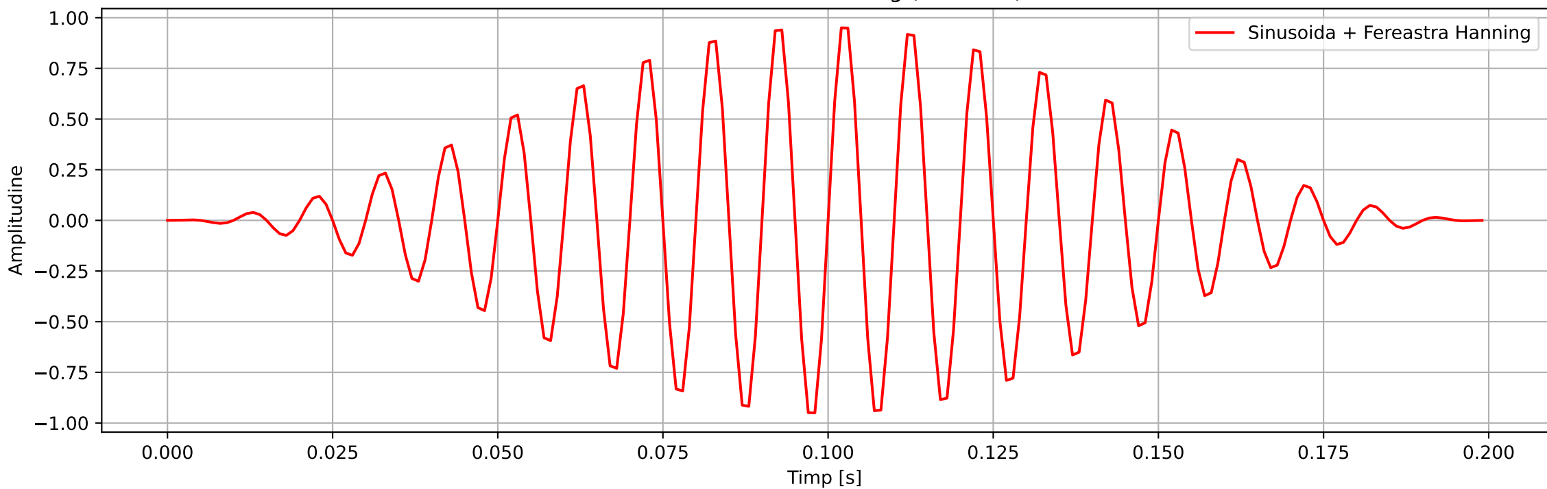
Efectul Ferestrei Hanning (f=100Hz)
